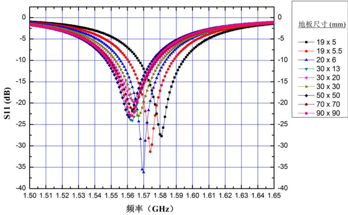
地板尺寸对频率的影响
